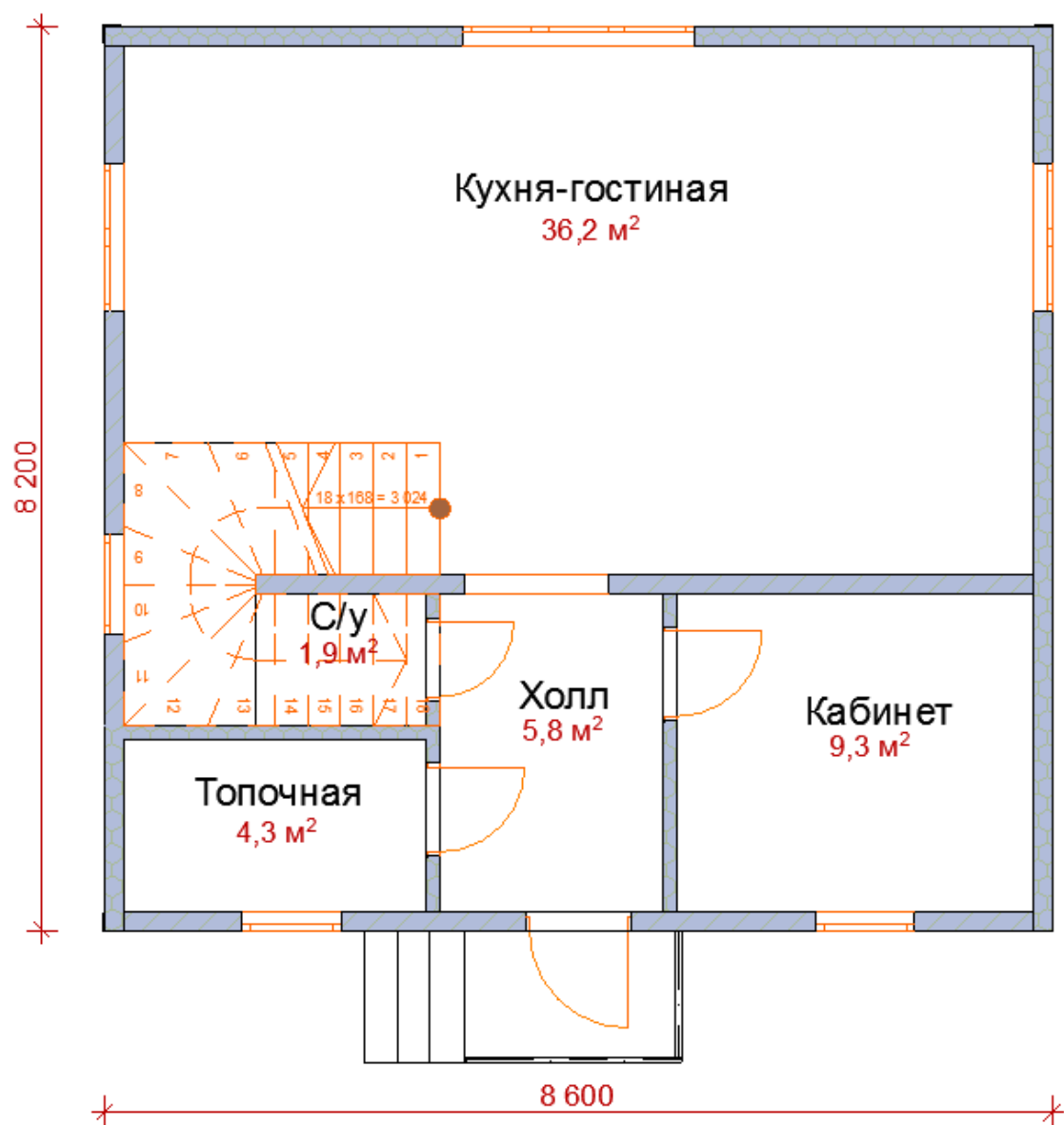
Первый этаж
