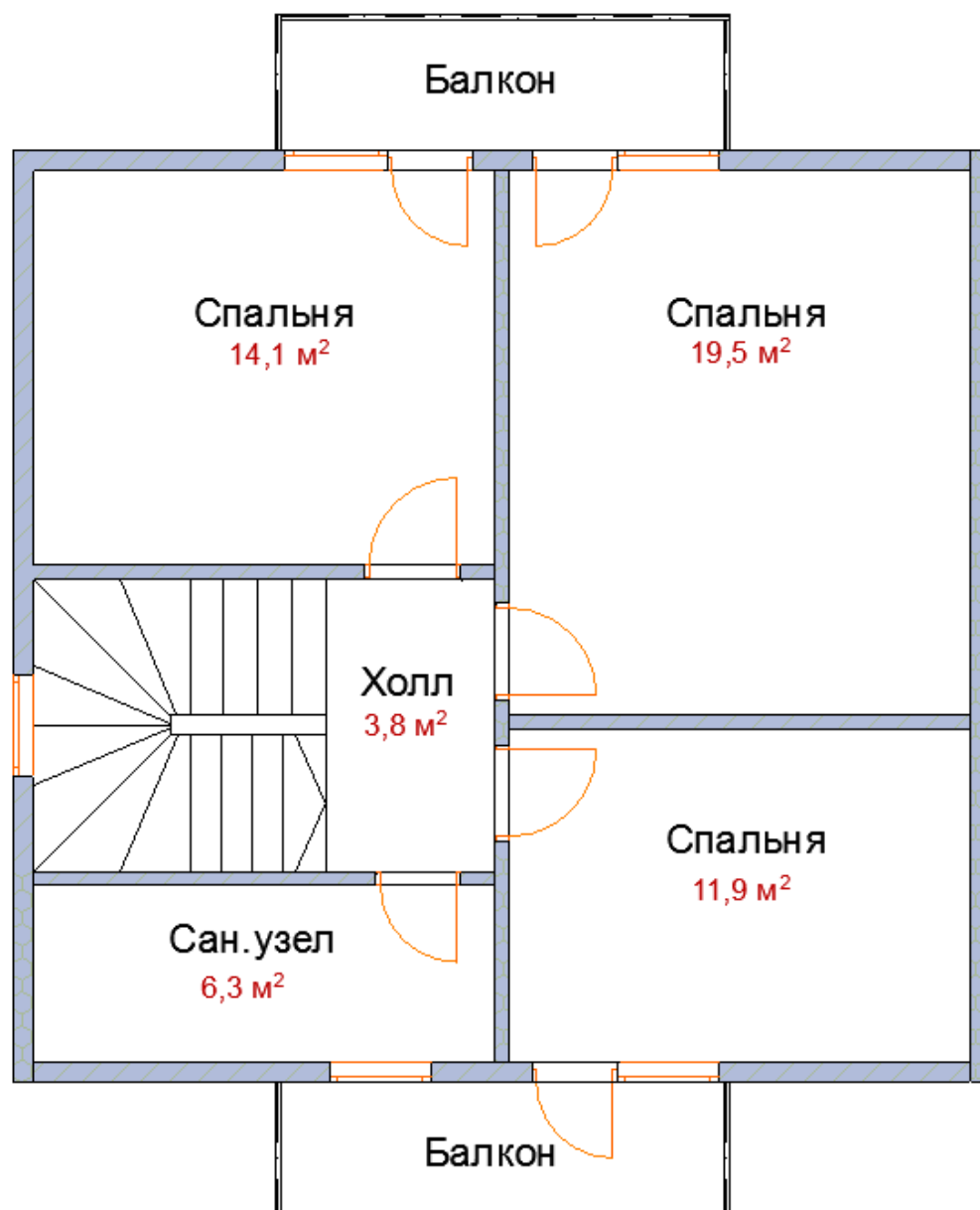
План мансарды
