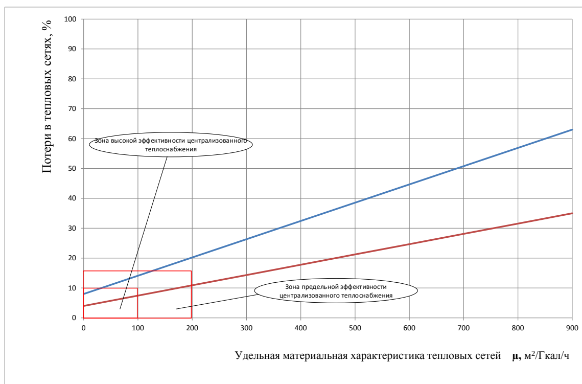
Рис. 3. Зависимость потерь тепловой энергии в тепловых сетях от удельной материальной характеристики тепловых сетей
