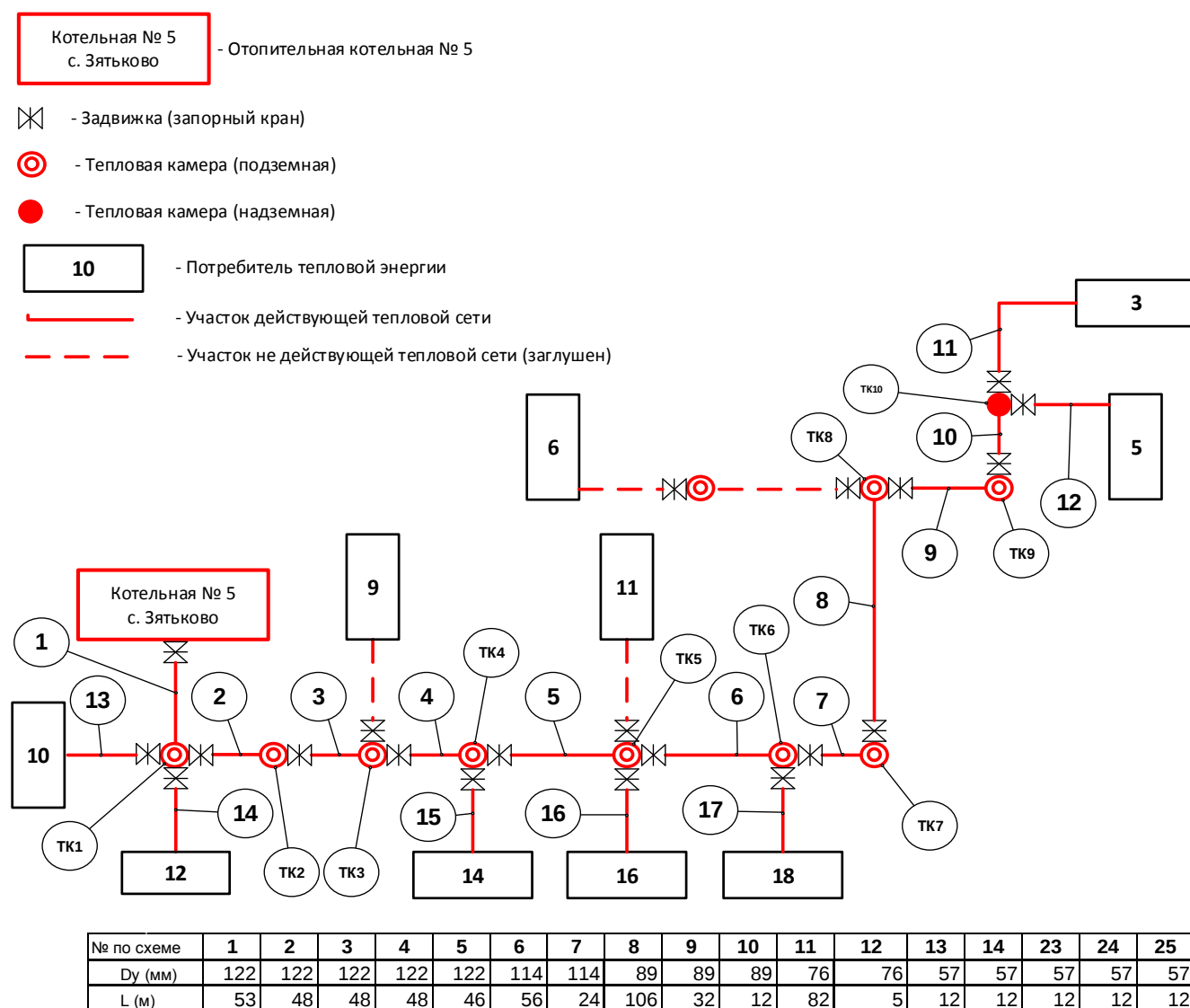
Рис. 4. Зоны теплоснабжения котельной № 5 с. Зятыково.
